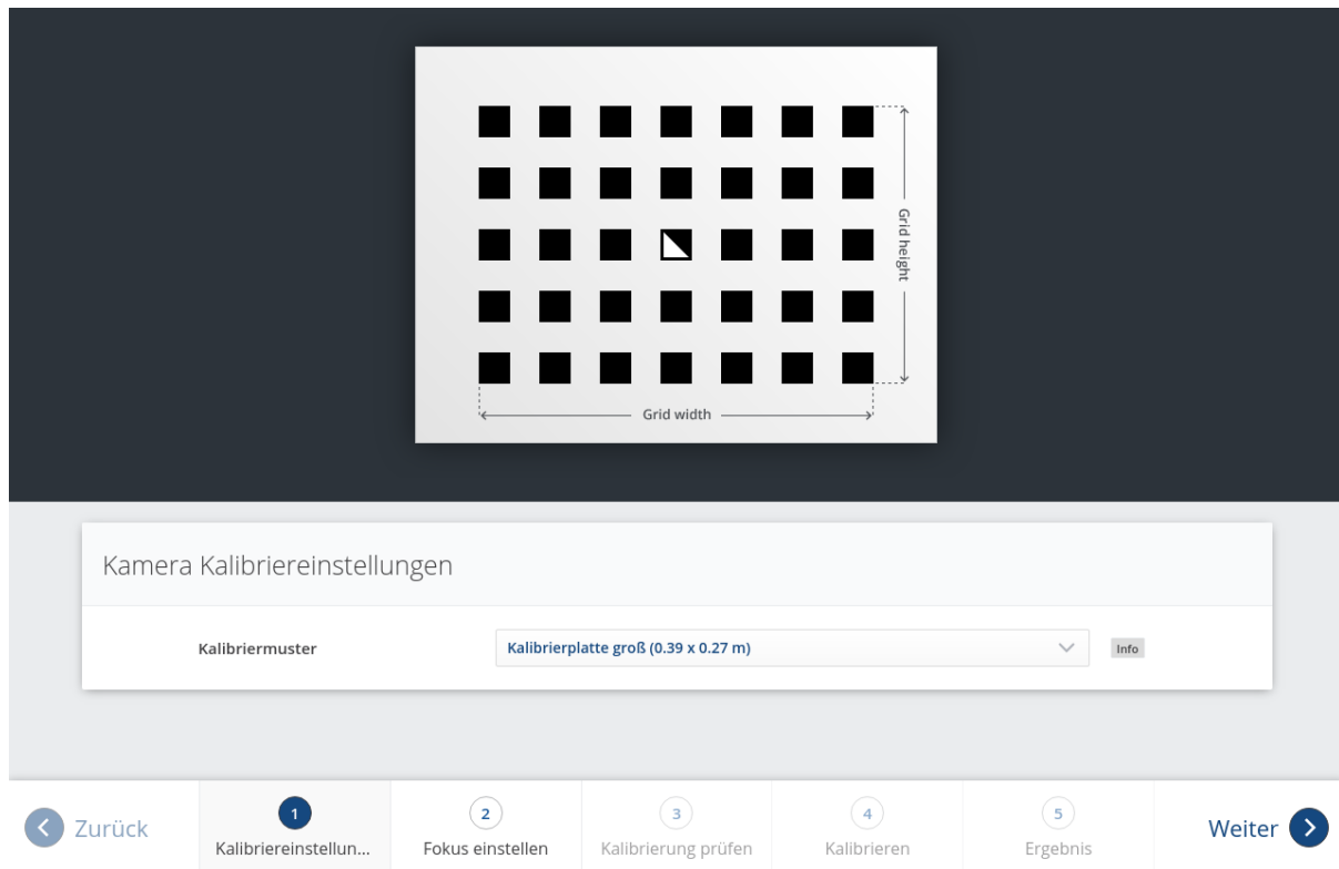
Abb. 6.26: Kalibriereinstellungen
