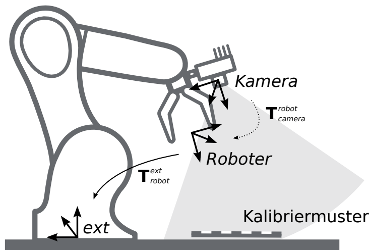
Abb. 6.15: Wichtige Koordinatensysteme und Transformationen für die Kalibrierung einer robotergeführten Kamera: Sie wird mit einer festen relativen Position zu einem benutzerdefinierten Roboter-Koordinatensystem (z.B. Flansch oder Werkzeugmittelpunkt) montiert. Es ist wichtig, dass die Pose T_{\text{robot}}^{\text{ext}} des Roboter-Koordinatensystems in Bezug auf ein benutzerdefiniertes externes Referenzkoordinatensystem (ext) während der Kalibrieroutine gemessen werden kann. Das Ergebnis des Kalibriervorgangs ist die gewünschte Kalibriertransformation T_{\text{camera}}^{\text{robot}} , d.h. die Pose des Kamera-Koordinatensystems im benutzerdefinierten Roboter-Koordinatensystem.
