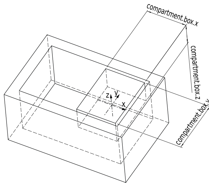
Abb. 6.40: Beispiel für ein Abteil innerhalb eines Load Carriers. Das gezeigte Koordinatensystem das Koordinatensystem des Load Carrier Abteils.
