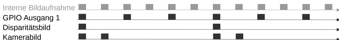
Abb. 6.35: Beispiel für die Nutzung der Betriebsart ExposureAlternateActive für GPIO-Ausgang 1 mit einer benutzerdefinierten Bildwiederholrate von 8 Hz. Die interne Bildaufnahme geschieht immer mit 25 Hz. GPIO-Ausgang 1 ist für die Dauer der Belichtungszeit jedes zweiten Bildes an (HIGH). Disparitätsbilder werden für Kamerabilder berechnet, bei denen GPIO-Ausgang 1 an (HIGH) ist, und die auch per GigE Vision in der benutzerdefinierten Bildwiederholrate versendet werden. In der Betriebsart ExposureAlternateActive werden Intensitätsbilder immer paarweise versendet: ein Bild mit GPIO-Ausgang 1 an (HIGH), für das ein Disparitätsbild verfügbar sein kann, und ein Bild mit GPIO-Ausgang 1 aus (LOW).
