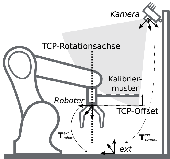
Abb. 6.19: Im Fall eines 4DOF-Roboters müssen die TCP-Rotationsachse und der Offset vom TCP zur sichtbaren Oberfläche des Kalibrier-musters entlang der TCP-Rotationsachse angegeben werden. Im dargestellten Fall ist der Offset negativ.
