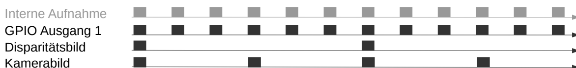
Abb. 6.34: Beispiel für die Nutzung der Betriebsart ExposureActive für GPIO-Ausgang 1 mit einer benutzerdefinierten Bildwiederholrate von 8 Hz. Die interne Bildaufnahme geschieht immer mit 25 Hz. GPIO-Ausgang 1 ist für die Dauer der Belichtungszeit jedes Bildes an (HIGH). Disparitätsbilder werden für Kamerabilder berechnet, die auch per GigE Vision in der benutzerdefinierten Bildwiederholrate versendet werden.
