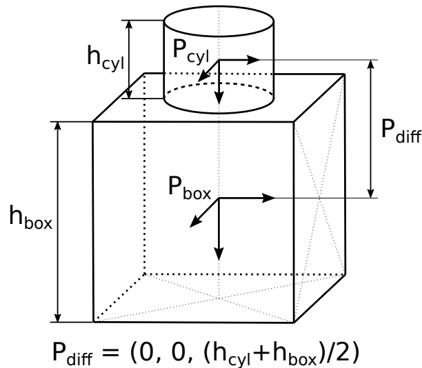
Abb. 6.45: Bezugskoordinatensysteme für das Erstellen von Greifern über die REST-API und die Web GUI
