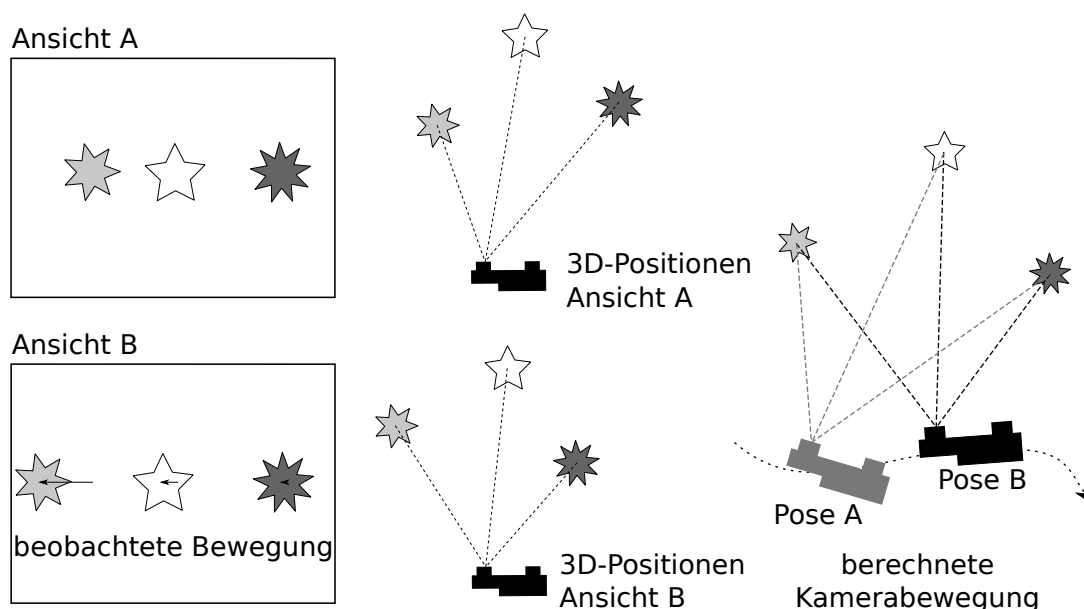
Abb. 5.3: Vereinfachte schematische Darstellung der stereobasierten visuellen Odometrie für 2D-Bewegungen: Die Kamerabewegung wird auf Grundlage der beobachteten Bewegung charakteristischer Bildpunkte berechnet.
