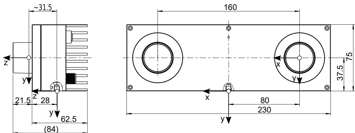
Abb. 3.10: Ungefähre Position des Sensor-/Kamerakoordinatensystems (in der linken Kameralinse) und des Montagepunkt-Koordinatensystems (am Stativgewinde) für den rc_visard 160
